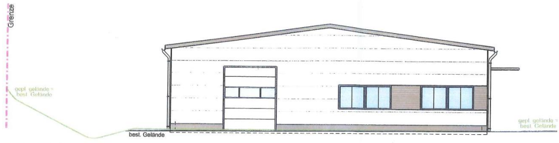
Ostansicht
