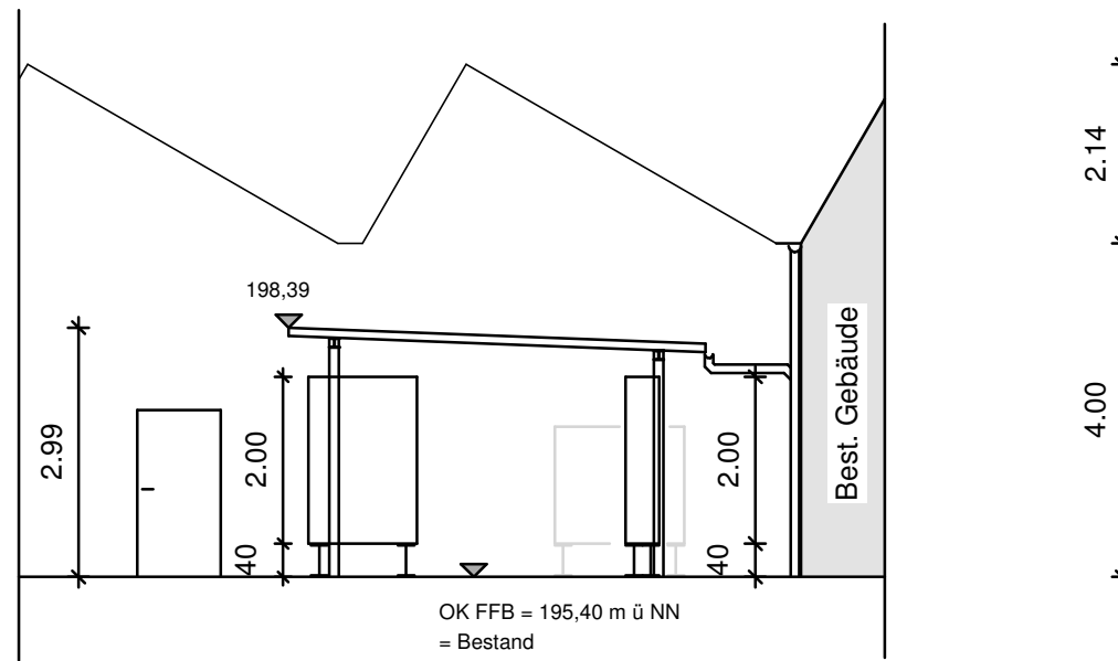
Ansicht WEST
