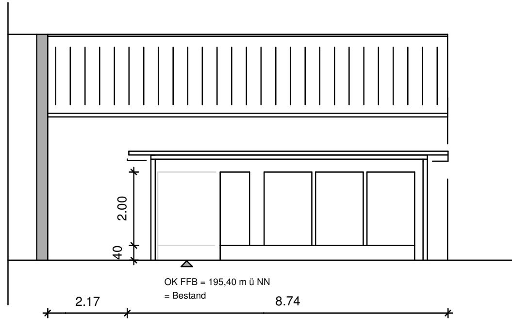
Ansicht SÜD
