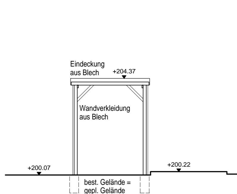
SCHNITT A-A
