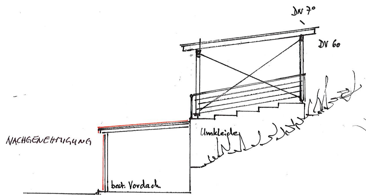
Ansicht Norden
