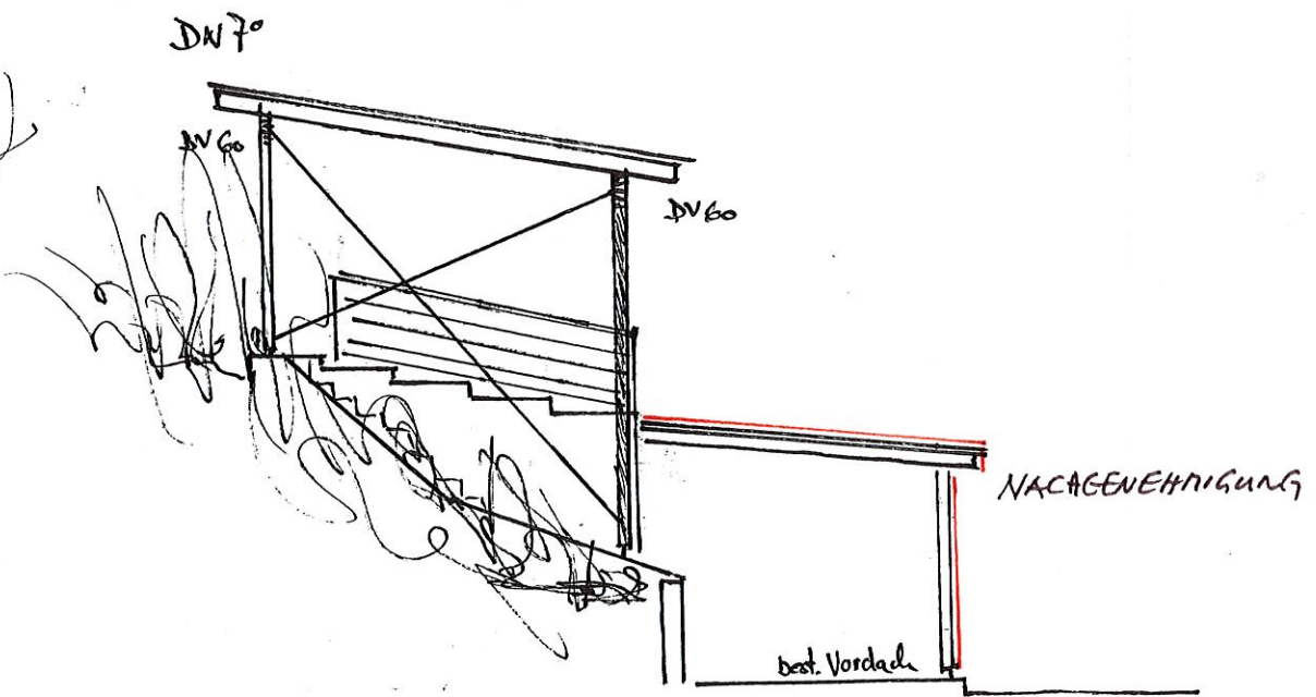
Ansicht Süden
